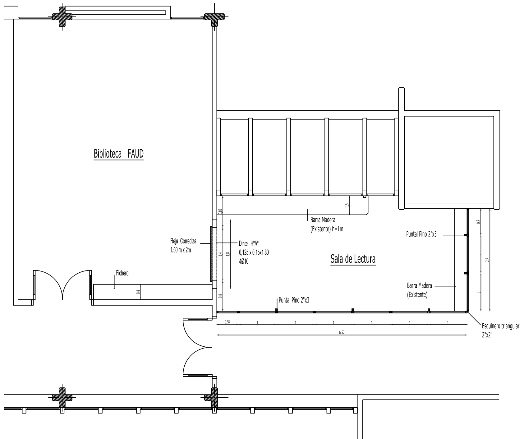
PLANTA - Nivel 4
