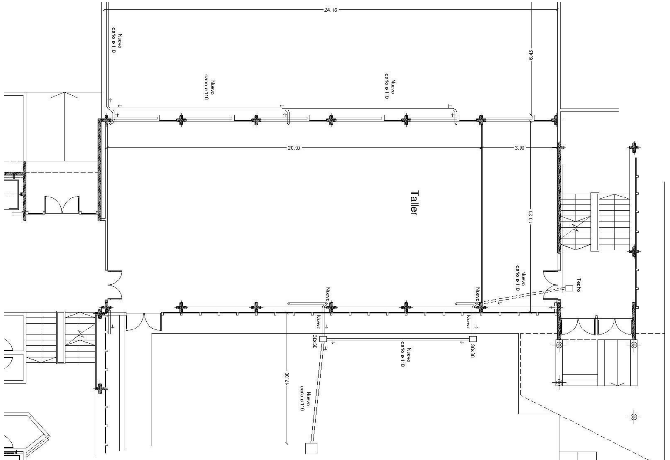
Desagües existentes a reemplazar en taller 4 de Arquitectura
