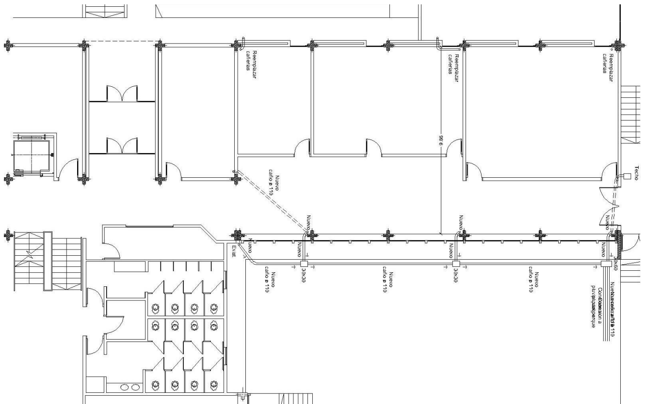
Esquema de desagües a realizar a nuevo de taller 6 de Arquitectura
